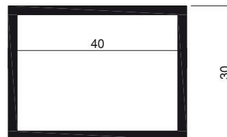
Art.Nr. A9430 RR - Hohlprofil 30x40x2
