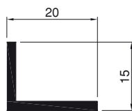
Art.Nr. A8215 L - Winkelprofil 20x15x2
