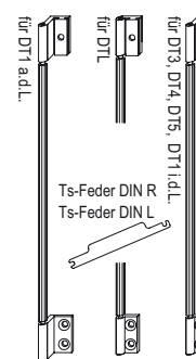
Art.Nr. B460 Schließhilfe für Drehtür Beschlagsatz 4-teilig
