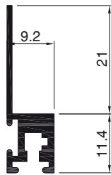
Art.Nr. A7010 h - Bürstenführungsprofil
