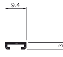
Art.Nr. A7030 c - Bürstenführungsprofil
