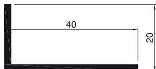
Art.Nr. A8420 L - Winkelprofil 40x20x2
