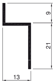
Art.Nr. A7060 Z - Profil Befestigungsschiene für Spannrahmen
