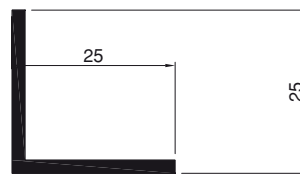
Art.Nr. A8225 L - Winkelprofil 25x25x2
