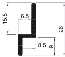
Art.Nr. A1350 Z - Profil Führungsschiene für Schiebetüre
