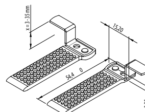
Art.Nr. B230 Mittelarretierung
