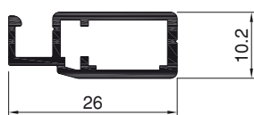
Art.Nr. A1010 Spannrahmenprofil
