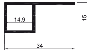
Art.Nr. A1570 Einbaurahmenprofil
