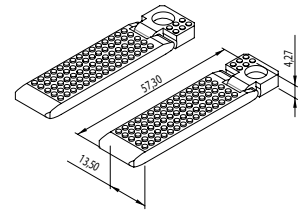
Art.Nr. B612 Klappgriff
