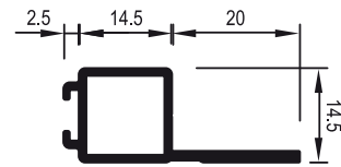
Art.Nr. A1470 Einbaurahmenprofil mit Falz für Duplextür
