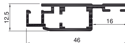
Art.Nr. A1230 Drehrahmenprofil mit Falz innen
