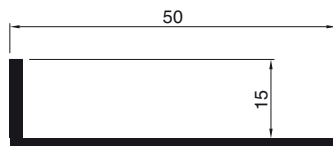
Art.Nr. A8515 L - Winkelprofil 50x15x2
